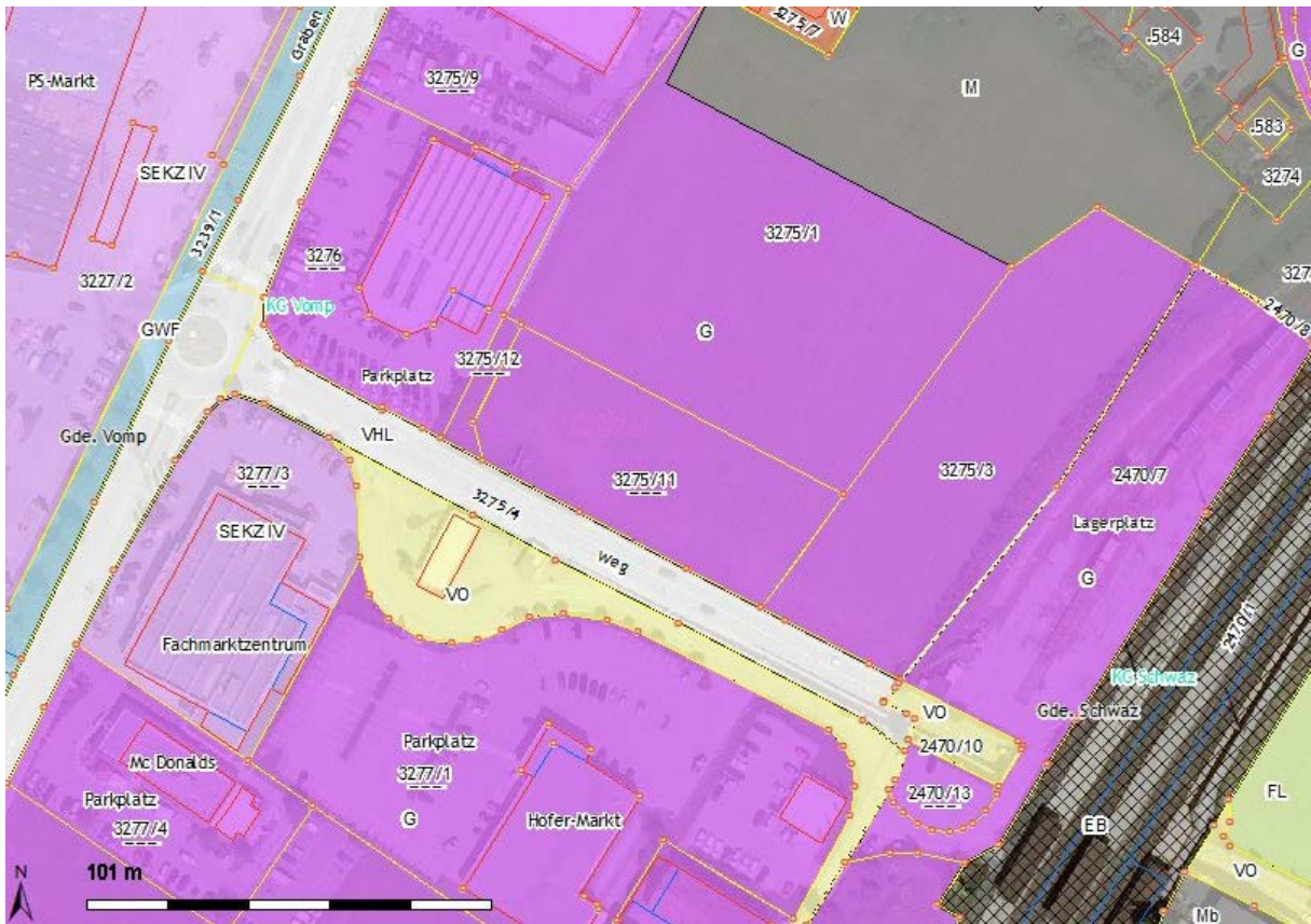
Flächenwidmungsplanauszug ©TIRIS – die Kaufflächen sind als Bauland-Gewerbe- und Industriegebiet (G) gewidmet
